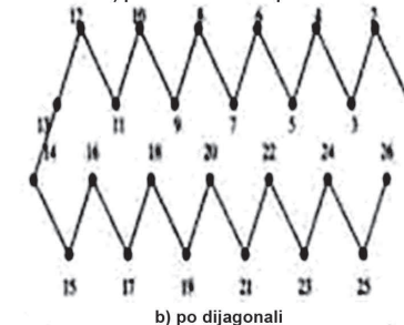
Način uzimanja uzoraka zemljišta na parceli a) po šahovskom rasporedu
